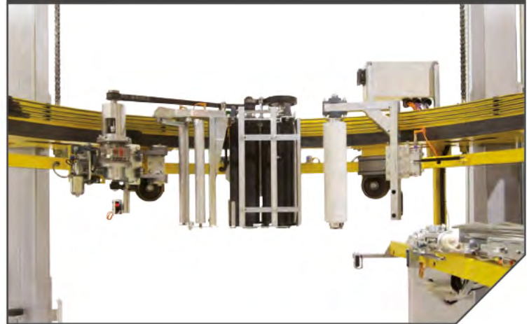
GRUPPO PRESTIRO FILM E CARRELLO PORTABOBINA (BREVETTATO MECWRAP) FILM PRE-STRETCHING AND REEL-HOLDER CARRIAGE UNIT (PATENTED) UKŁAD WSTĘPNEGO ROZCIĄGU FOLII STRETCH (OPATENTOWANY) FOLIENVORRECKUNG UND FOLIENWAGEN (MECWRAP-PATENT)
